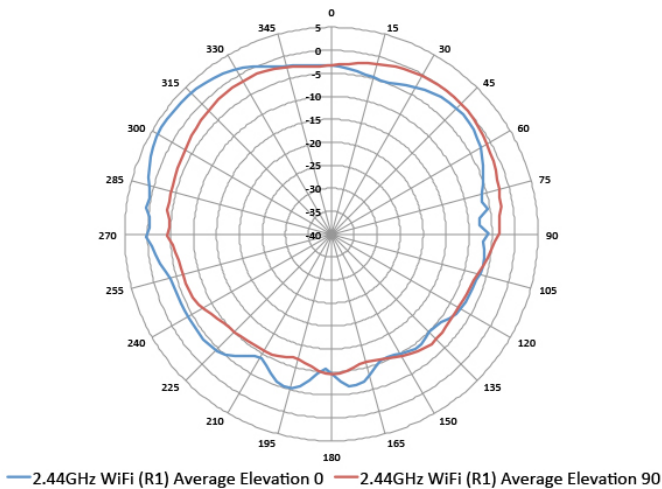
2.44GHz Wi-Fi (antennas 1, 2)
